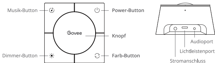
Steuerbox
