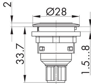
Maßskizze:
