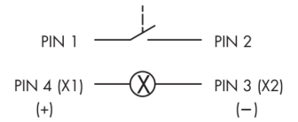
Schaltbild:
