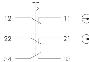
Schaltbild:
